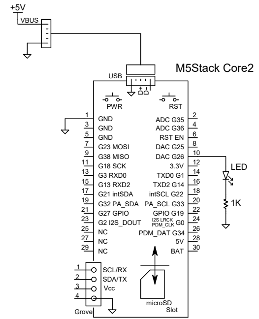
M5Stack Core2 Lチカ 電気回路図
